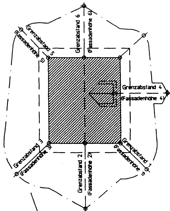
Grenzabstand im Verhältnis der Fassadenhöhe
